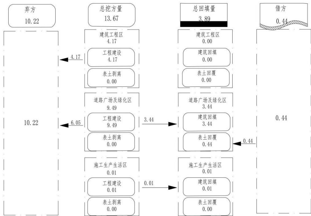
图2.4-1土石方平衡流向框图
